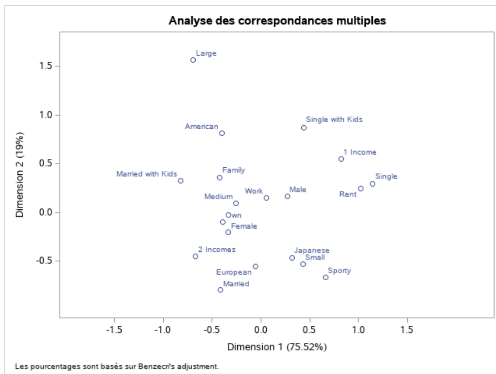
Figure 167 – Représentation des modalités dans le premier plan – Données "Cars"
