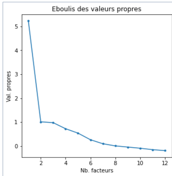
Figure 74 – Eboulis des valeurs propres – AFP – Données "Autos bruitées"
