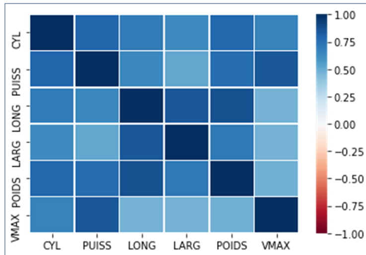
Figure 7 – "Heatmap" des corrélations croisées – Données "Autos"
