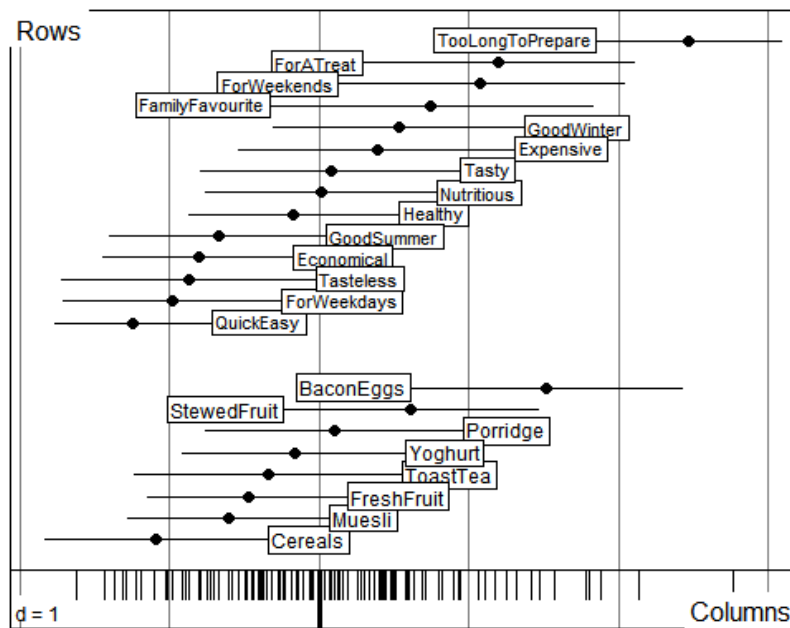
Figure 140 – Variante de la représentation simultanée – AFC – R, package "ade4"
