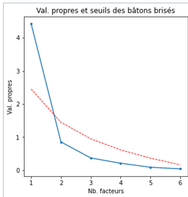
Figure 10 – Valeurs propres et seuils des bâtons brisés – Données "Autos"
