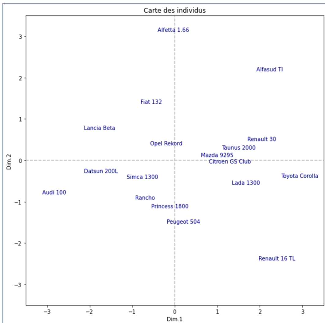
Figure 58 - Carte des individus - ACP sur corrélations partielles
