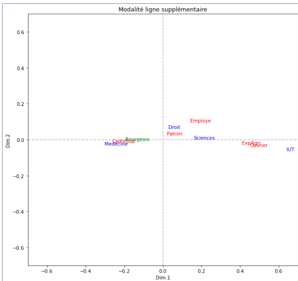
Figure 120 – Position de la modalité supplémentaire dans le plan factoriel – Données "CSP Filières"
