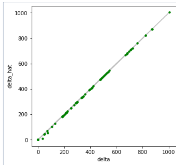
Figure 90 – Diagramme de Shepard – MDS – Données "Autos-MDS"
