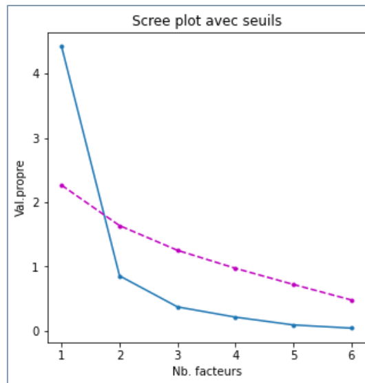
Figure 43 – Eboulis des v.p. et seuils d'acceptation – Données "Autos"
