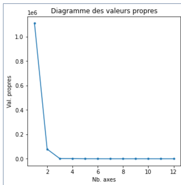
Figure 88 – Eboulis des valeurs propres – MDS – Données "Autos-MDS"
