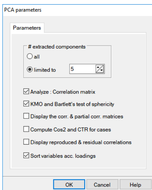
Figure 27 – Boîte de paramétrage – Principal Component Analysis – TANAGRA
