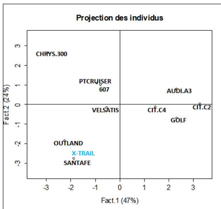
Figure 190 – Individu supplémentaire – AFDM – Données "Autos 2005"
