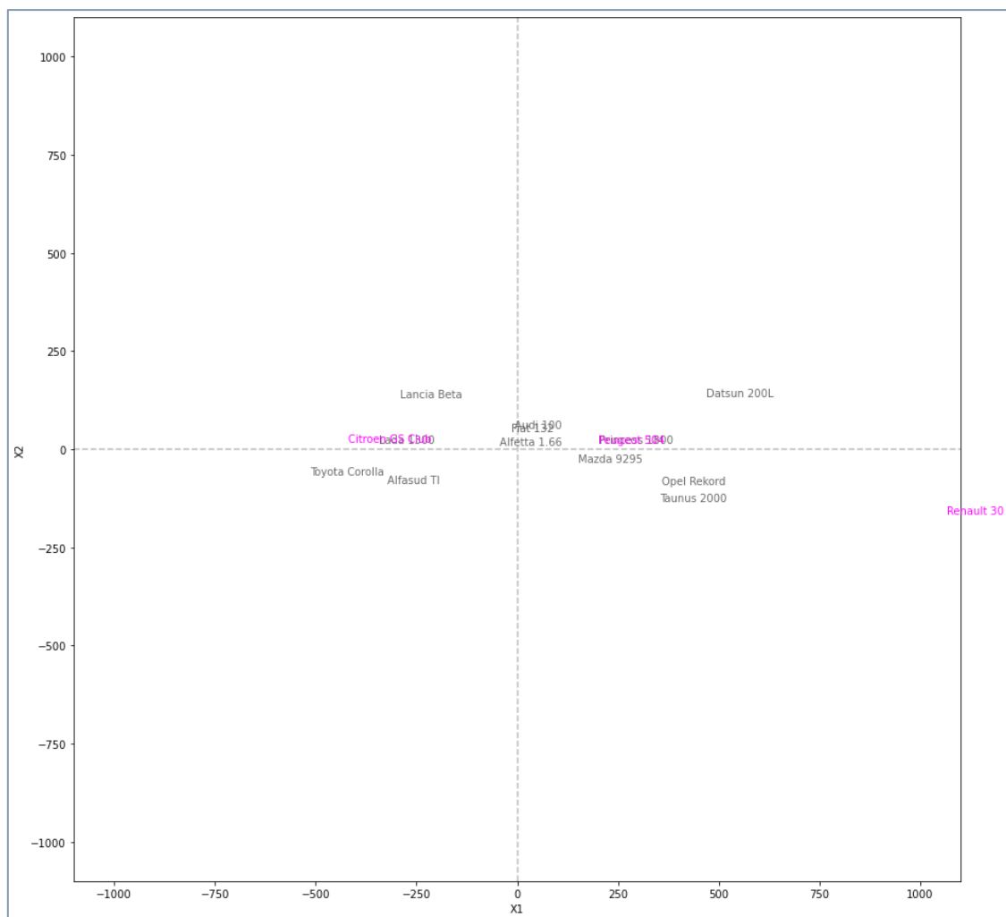
Figure 92 – Position des individus supplémentaires (magenta) – Données "Autos-MDS"
