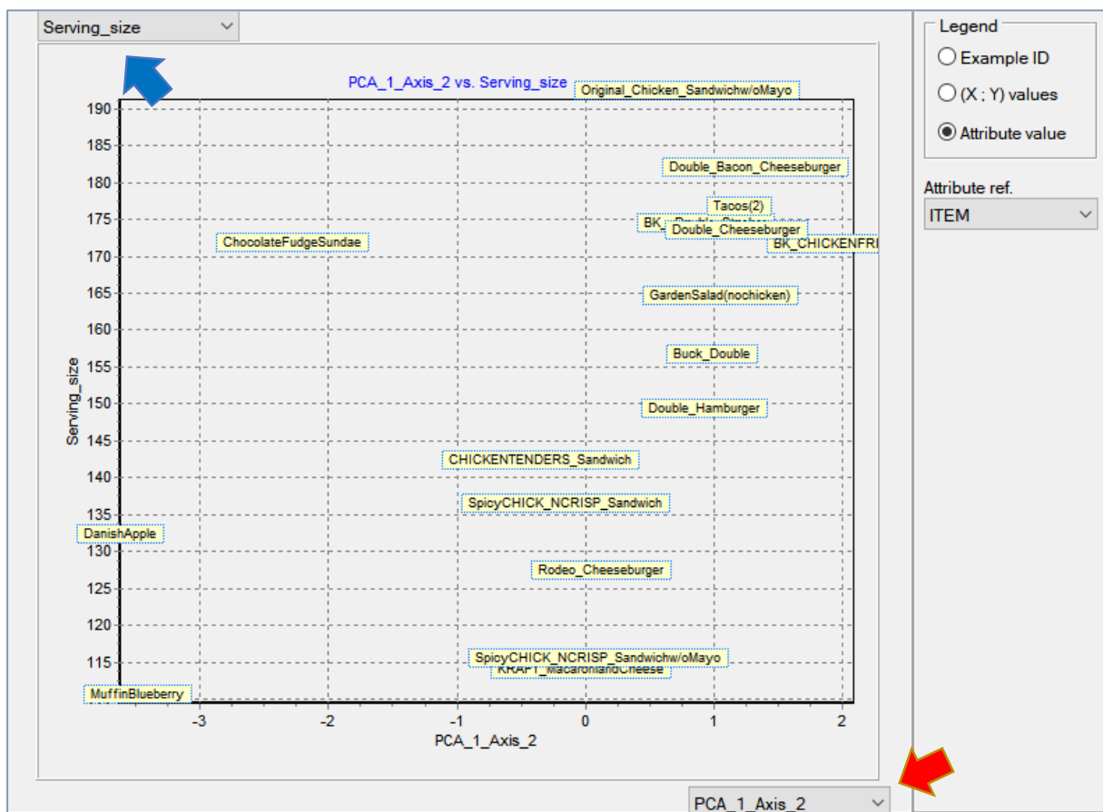
Figure 35 – Représentation des individus – 2nd facteur vs. Servig Size – TANAGRA
