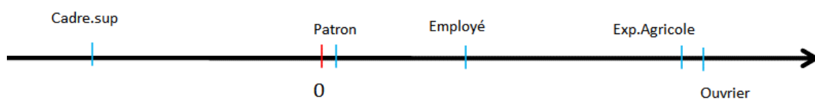
Figure 104 – Position des modalités lignes sur le 1er facteur de l'AFC - Données "CSP Filières"
