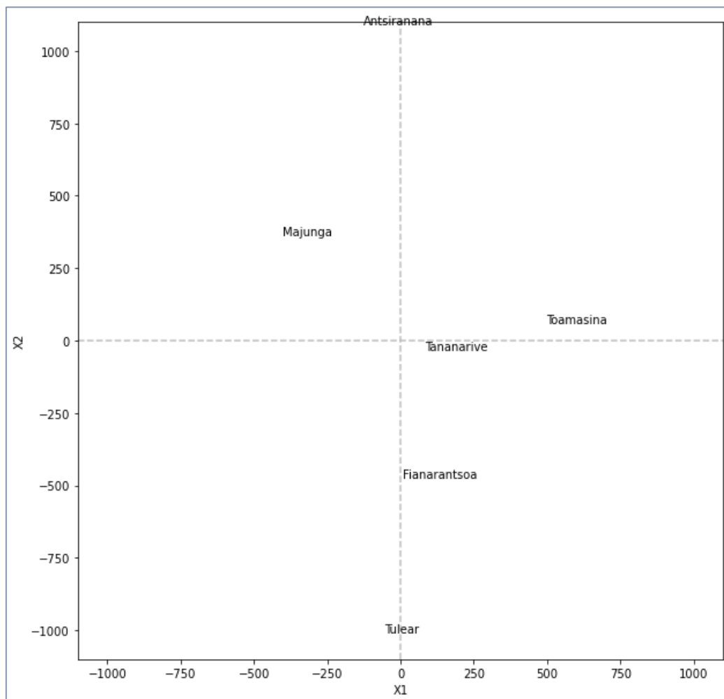
Figure 96 – Représentation des villes de Madagascar dans le plan – MDS
