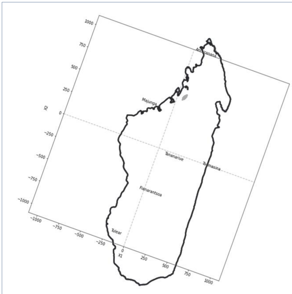
Figure 97 - Position des villes (MDS) et carte de Madagascar
