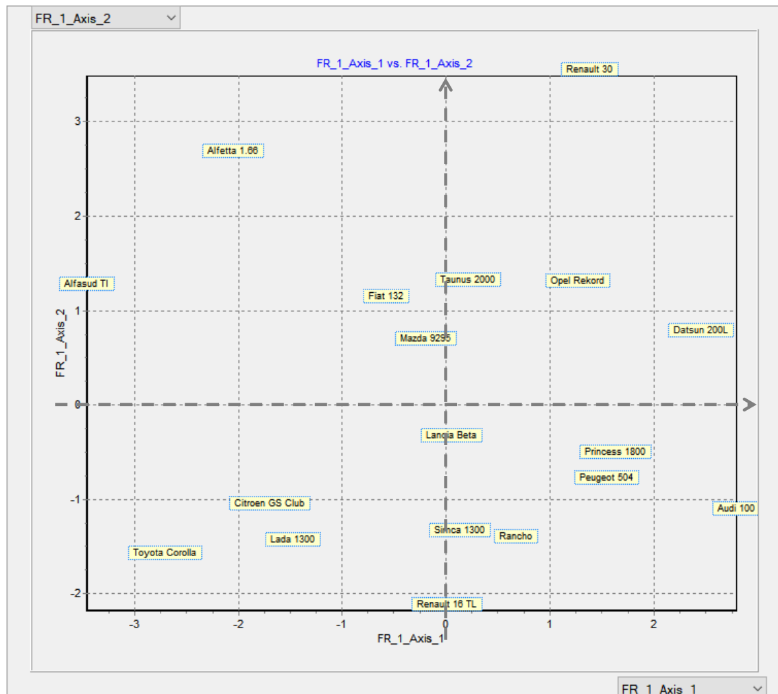
Figure 48 – Représentation dans le plan pivoté – Rotation VARIMAX – Données "Autos"
