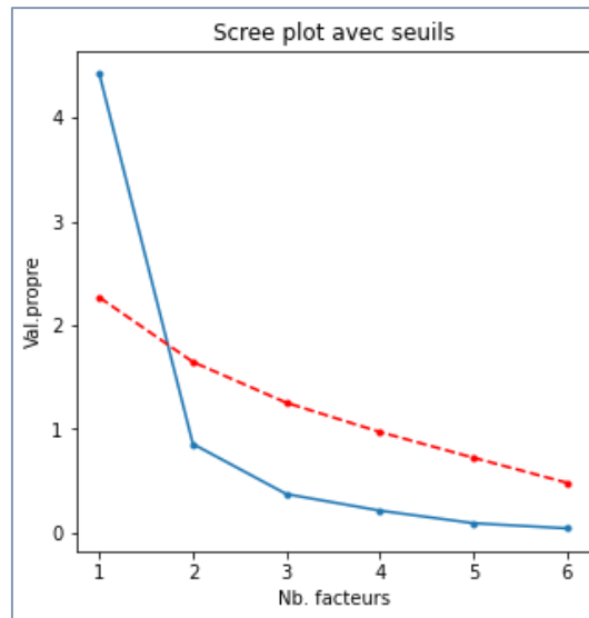
Figure 42 – Eboulis des v.p. et seuils de l'analyse parallèle – Données "Autos"
