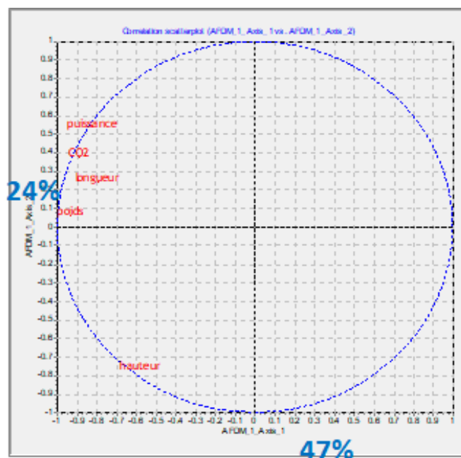
Figure 186 – Cercle des corrélations des variables quantitatives – AFDM – Données "Autos 2005"
