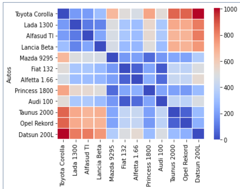
Figure 85 - "Heatmap" des distances entre paires d'individus - Données "Autos-MDS"
