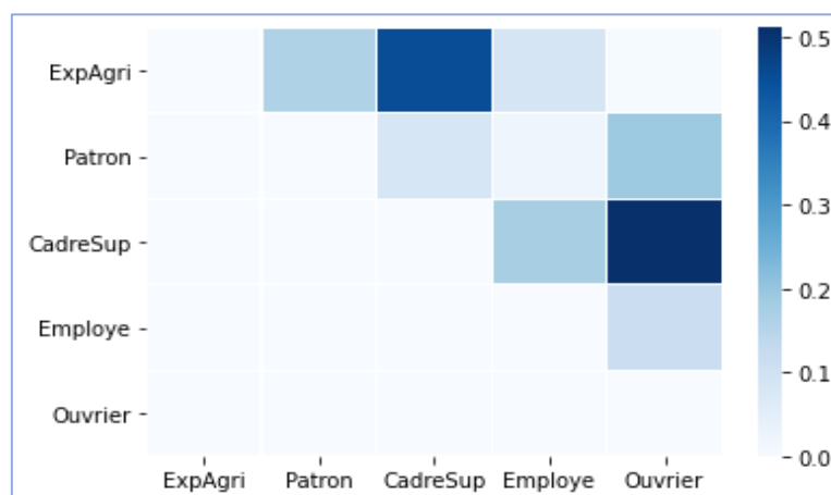
Figure 102 – Distances (au carré) entre les paires de modalités lignes – Données "CSP Filières"
