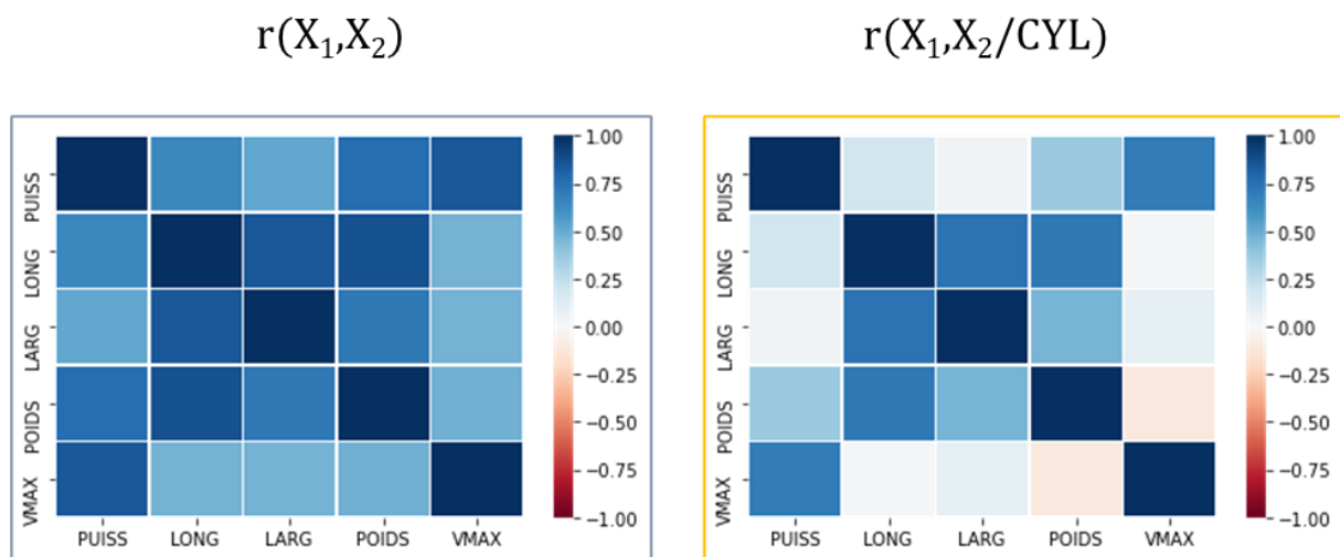
Figure 55 – Corrélations brutes et partielles relativement à CYL – Données "Autos"
