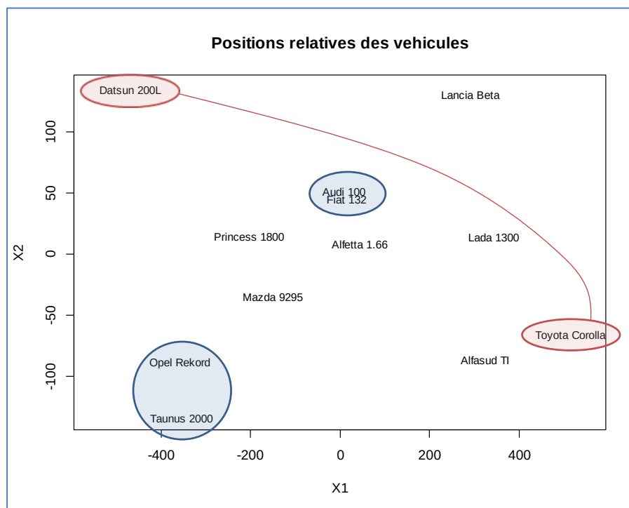
Figure 83 – Données "Autos-MDS" – Représentation dans le plan
