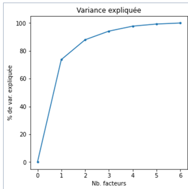
Figure 9 – Courbe de variance expliquée – Données "Autos"
