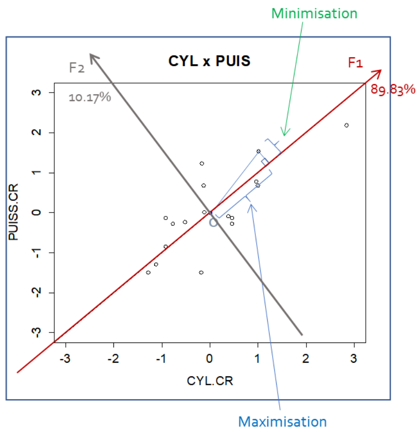
Figure 5 – Composantes principales – Données "Autos" (CYL, PUISS)
