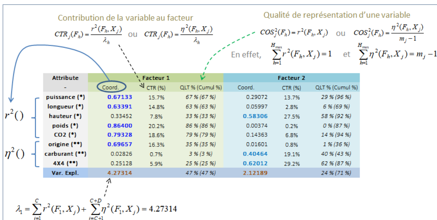
Figure 183 – Coordonnées des variables, contributions et COS2 – AFDM – Données "Autos 2005"
