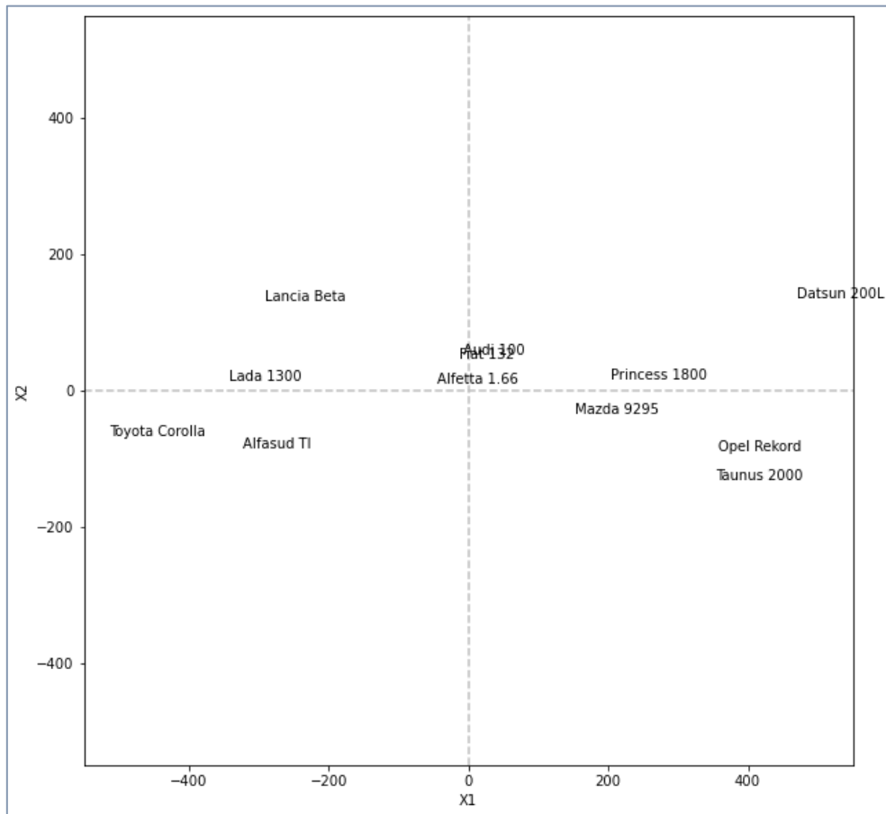
Figure 86 – Représentation des individus dans le plan – Données "Autos-MDS"
