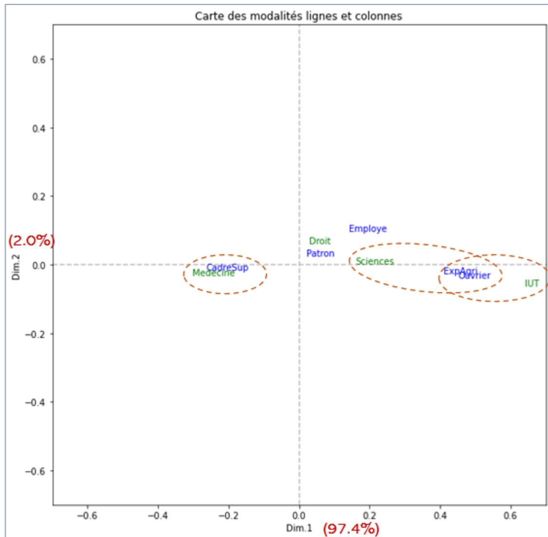
Figure 114 – Représentation simultanée dans le plan – Données "CSP Filières"
