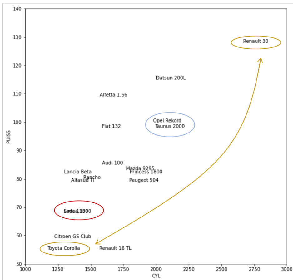
Figure 1 – ACP – Données "Autos" – Nuage de points (CYL vs. PUISS)
