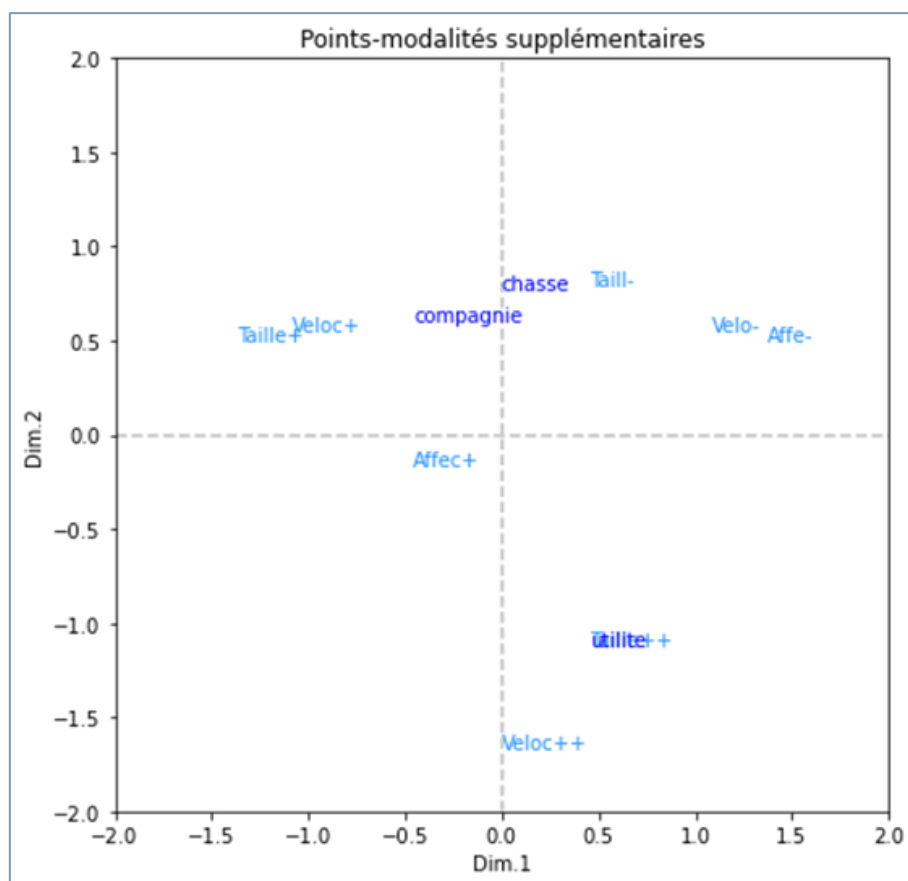
Figure 162 – Position des modalités de la variable illustrative "Fonction" – ACM – Données "Canidés"
