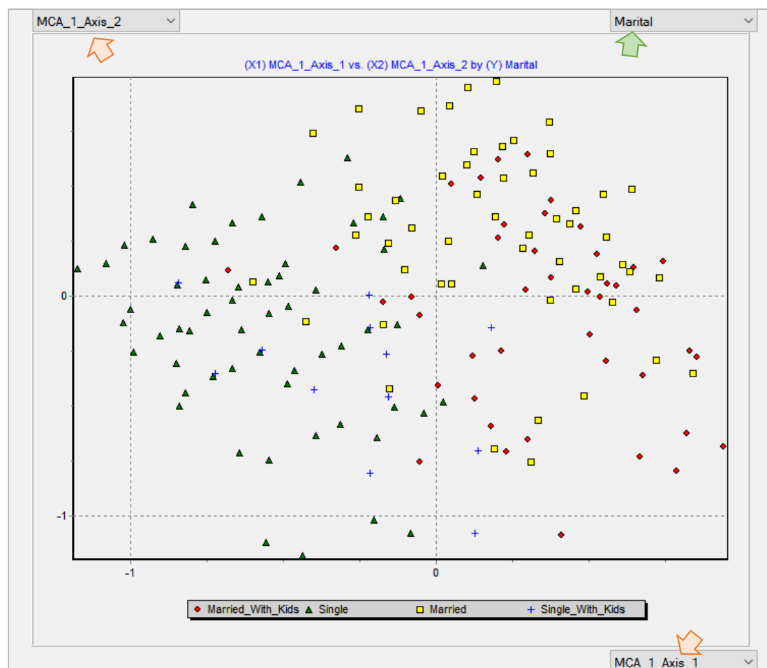
Figure 175 – Projection des individus dans (F1, F2) illustrés par "Marital" – TANAGRA – Données "Cars"
