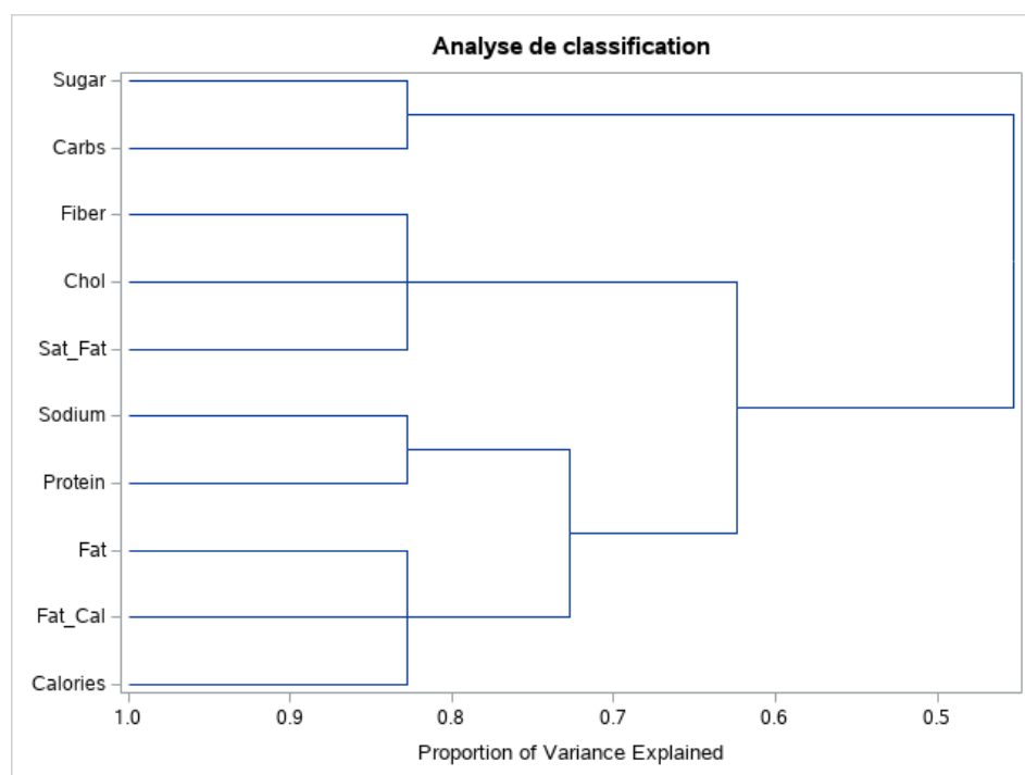
Figure 59 – Dendrogramme – VARCLUS – Données "Burger King"
