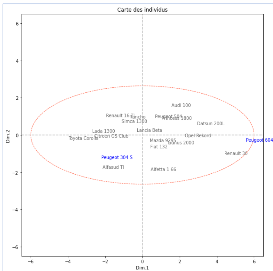
Figure 18 – Ellipse de confiance – Données "Autos"
