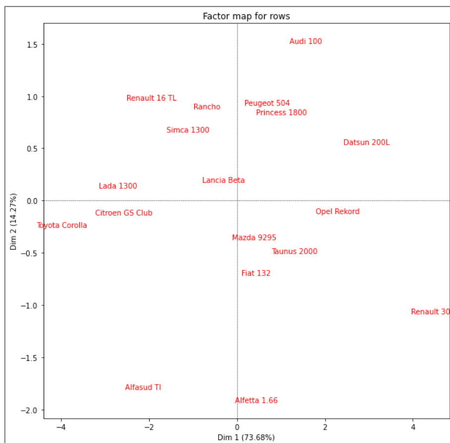
Figure 12 – Carte des individus – Version 1 – Données "Autos"
