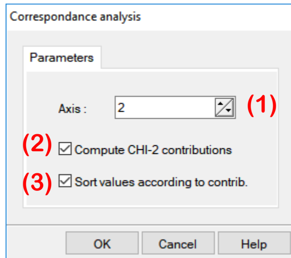
Figure 123 – Boîte de dialogue de paramétrage – AFC – Tanagra
