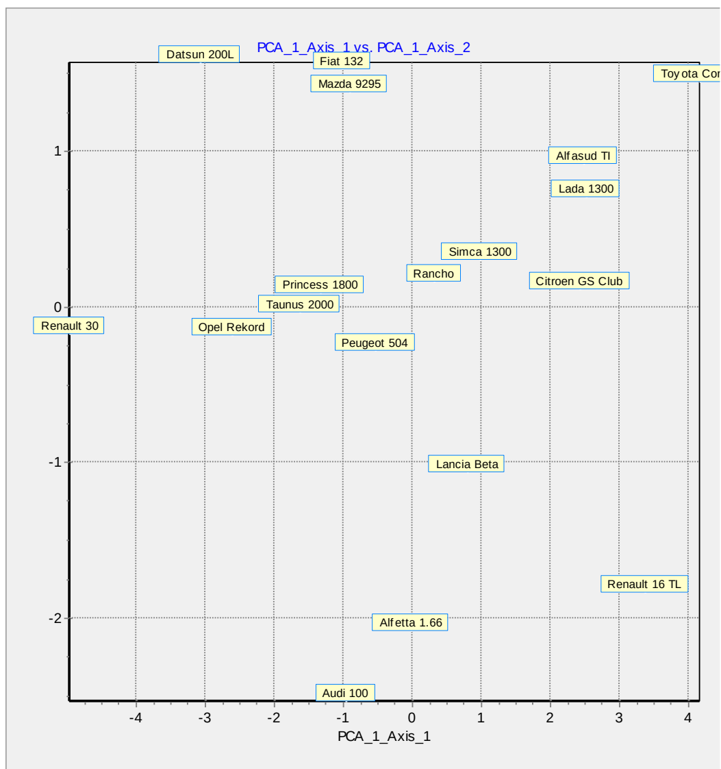
Figure 72 – Carte des individus – ACP – Données "Autos bruitées"
