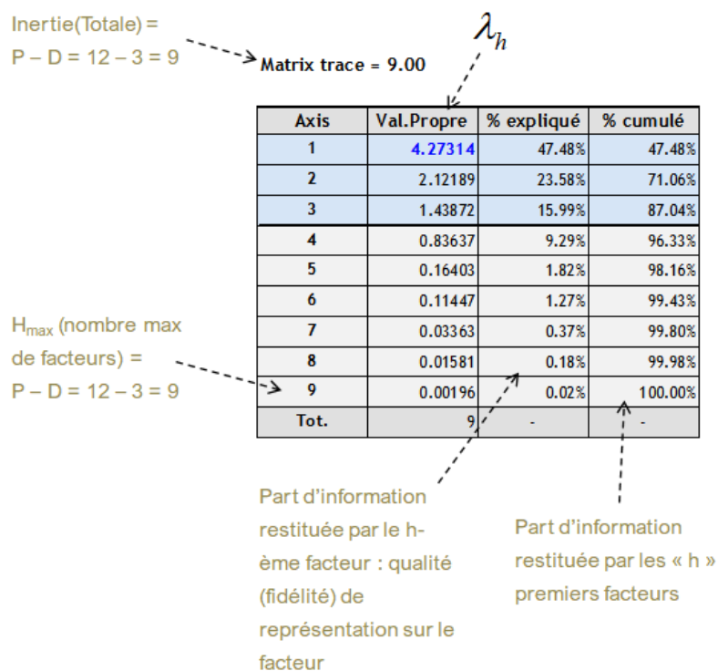
Figure 181 – Tableau des valeurs propres – AFDM – Données "Autos 2005"
