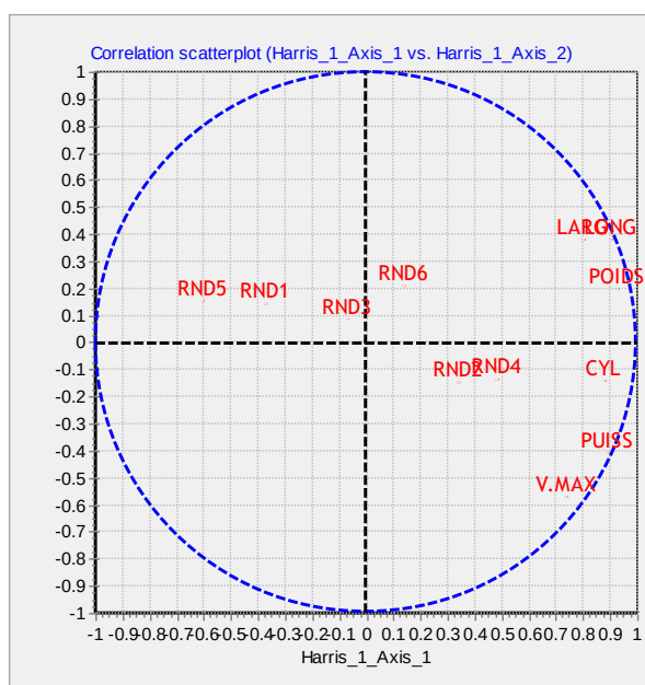
Figure 79 – Méthode de Harris – Cercle des « loadings » – Données "Autos bruitées"
