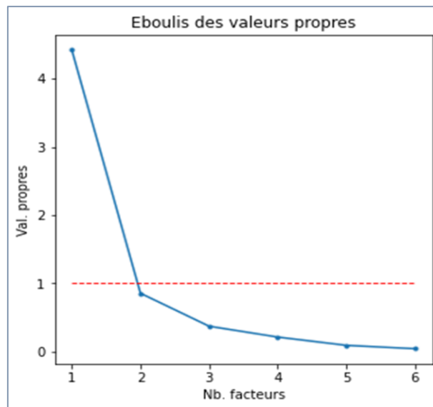
Figure 8 – Scree plot – Données "Autos"
