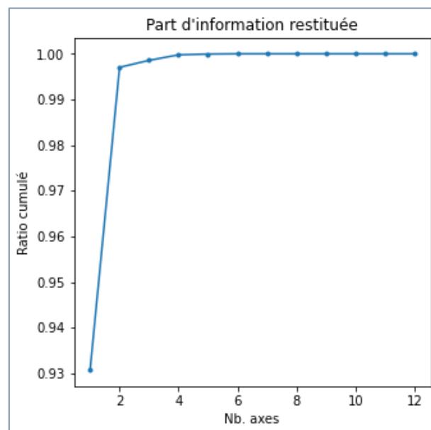
Figure 87 – MDS – Part d'information restituée par les "q" (q = 1 à 12) premiers axes – Données "Autos-MDS"
