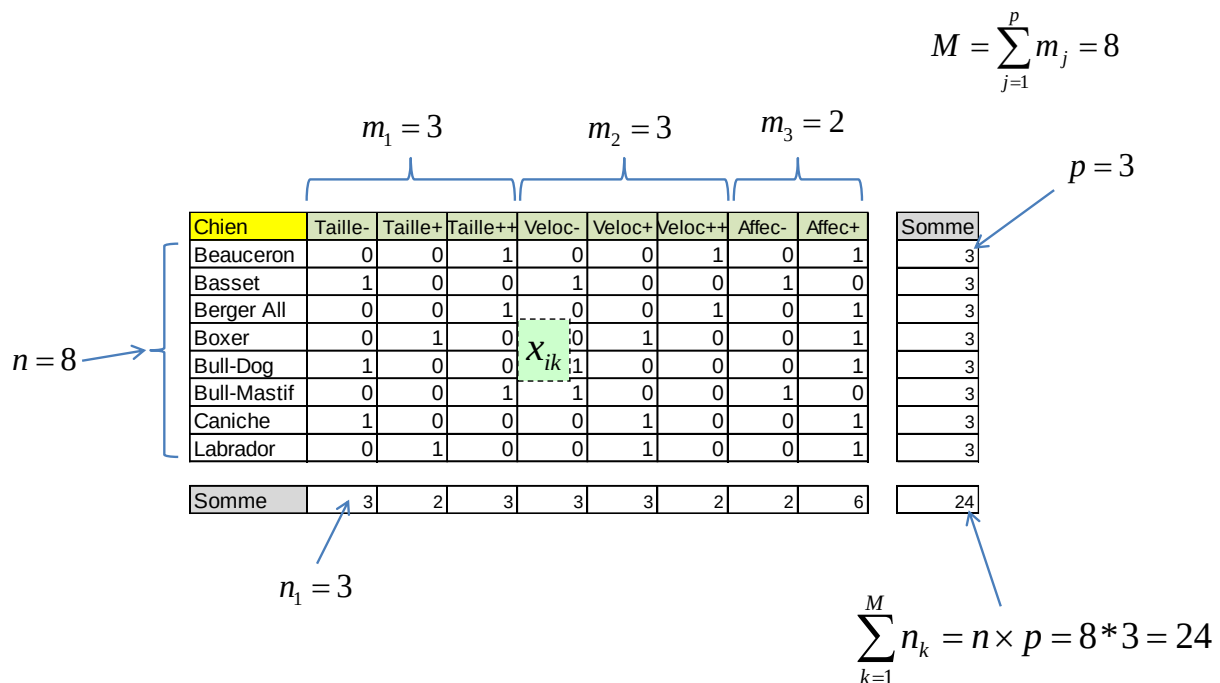
Figure 143 – Codage disjonctif complet – Notations
