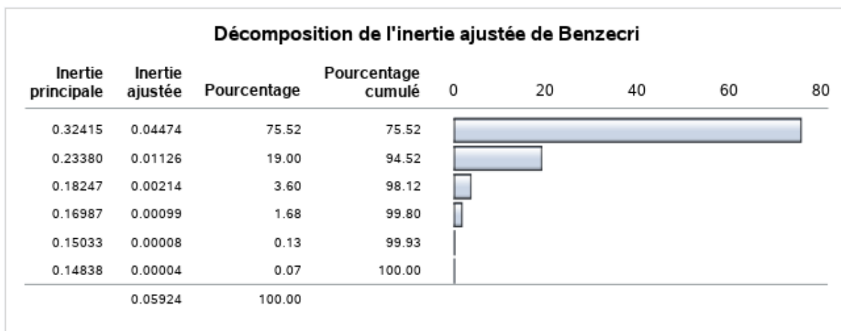
Figure 165 – Tableau des inerties – Proc Corresp – Données "Cars"
