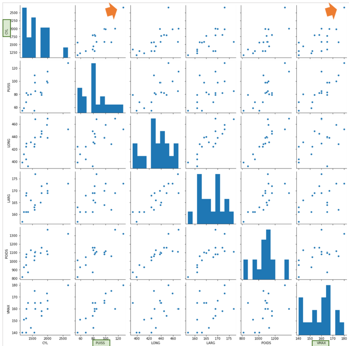
Figure 3 – ACP – Données "Autos" – Pairplot
