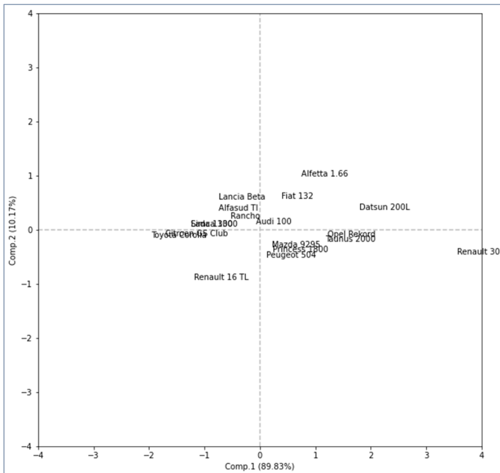
Figure 6 - Plan factoriel - Données "Autos" (CYL, PUISS)
