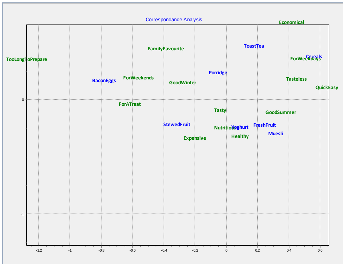
Figure 128 – Représentation simultanée – AFC – Tanagra
