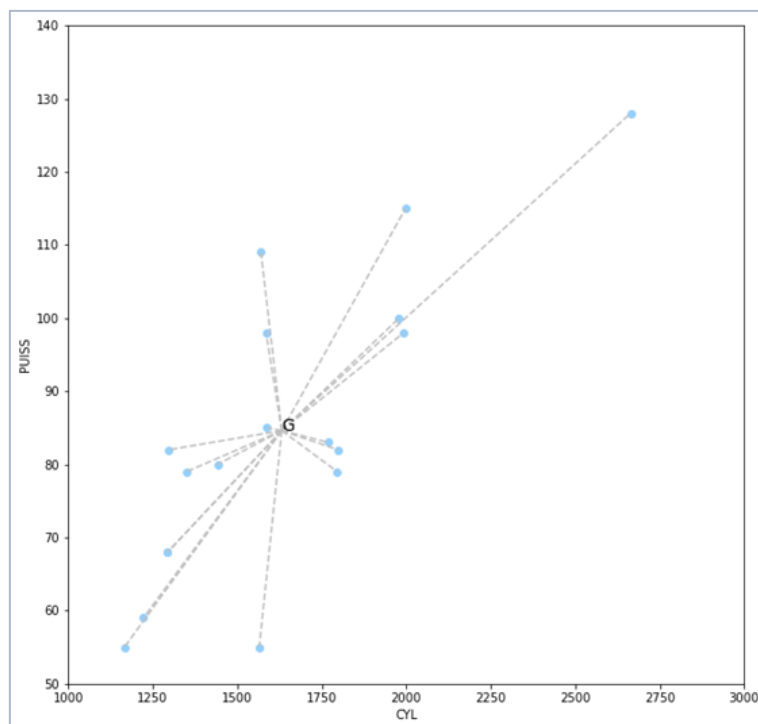
Figure 4 – Dispersion des points autour du barycentre G -- Données "Autos" (CYL, PUISS)
