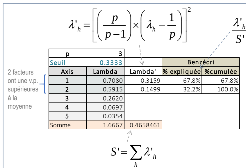
Figure 148 - Correction de Benzécri - ACM - Données "Canidés"
