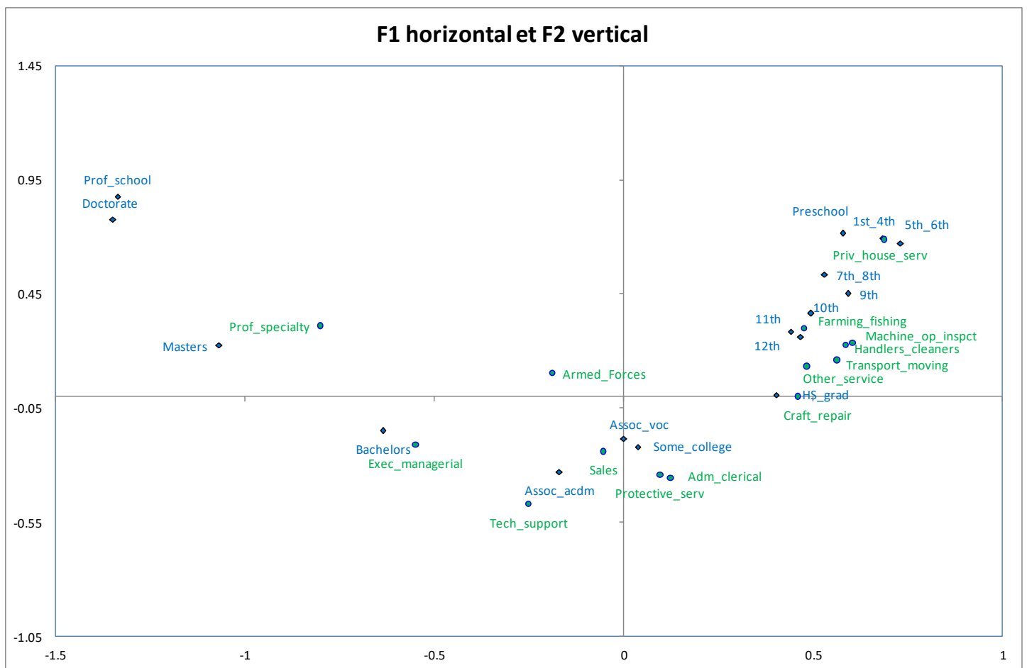
Figure 121 – Lien entre le niveau d'études et le type d'emploi occupé – TUTO 12
