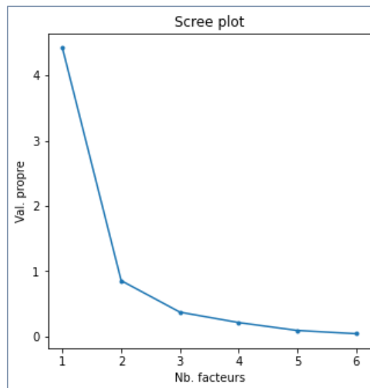
Figure 41 – Eboulis des v.p. – Données "Autos" – ACP normée
