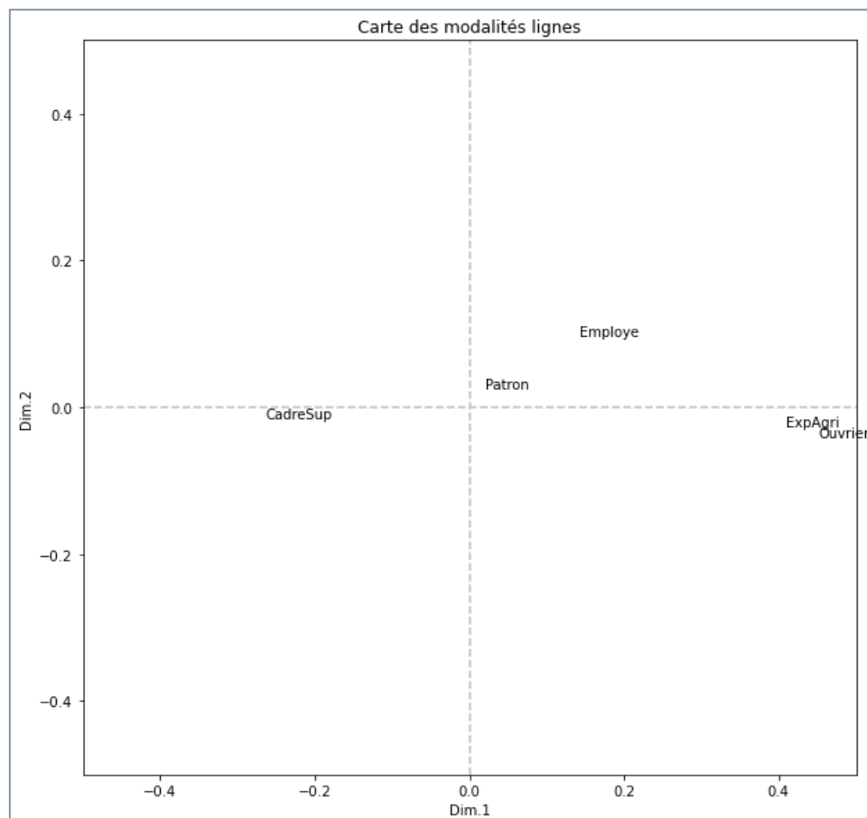
Figure 105 - Position des modalités lignes dans le plan - AFC - Données "CSP Filières"
