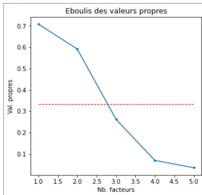
Figure 147 – Eboulis des valeurs propres – ACM – Données "Canidés"
