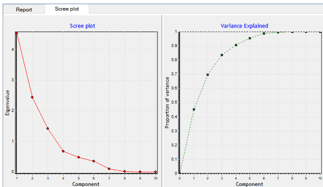
Figure 29 – Eboulis et prop. de variance expliquée – TANAGRA – Données "Burger King"
