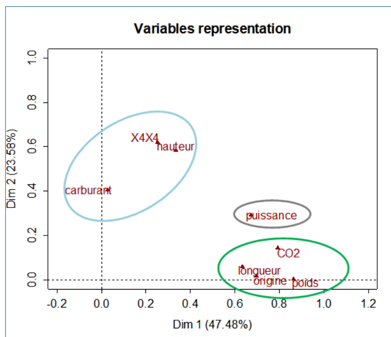
Figure 184 – Représentation des variables dans le 1er plan factoriel – AFDM – Données "Autos 2005"
