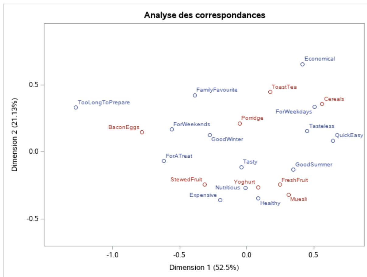
Figure 138 – Représentation simultanée – SAS PROC CORRESP
