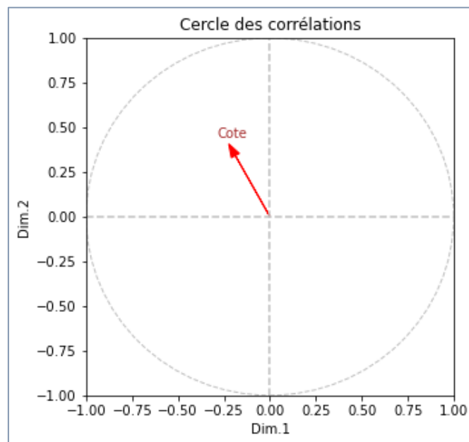
Figure 161 – Corrélations de la variable supplémentaire avec les facteurs (1, 2) – ACM – Données "Canidés"
