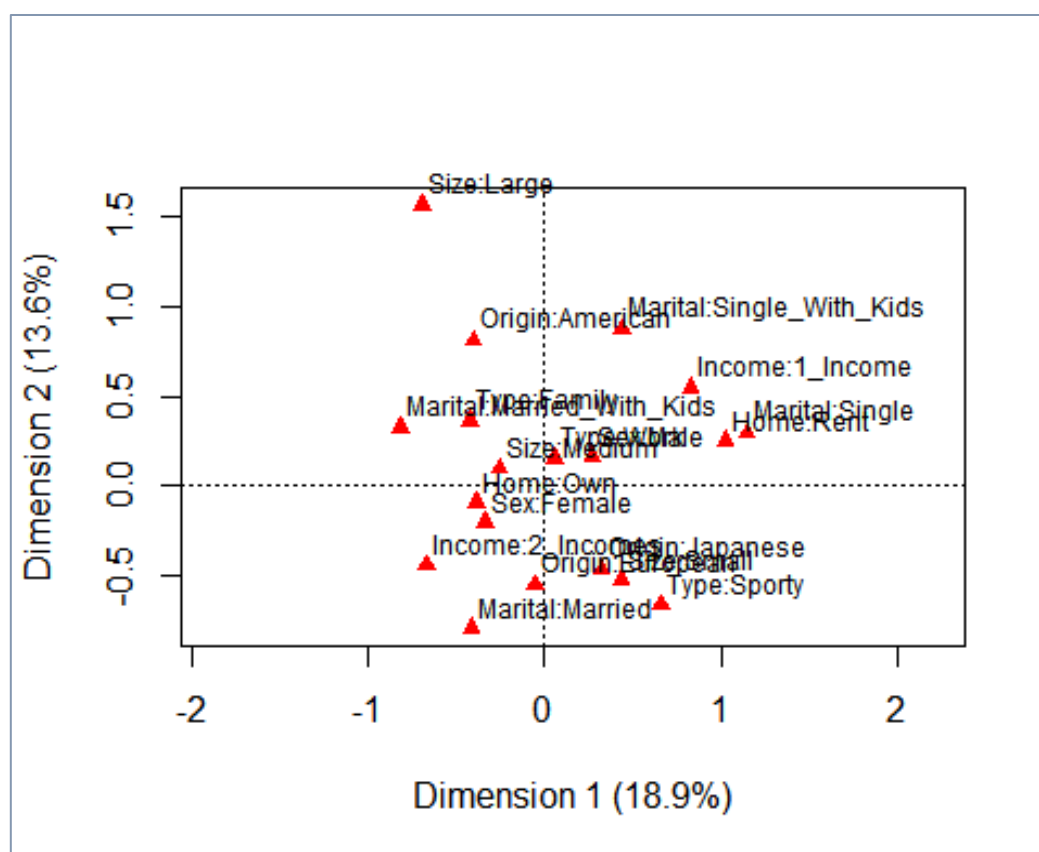
Figure 176 – Carte des modalités – ACM – R, package "ca" – Données "Cars"
