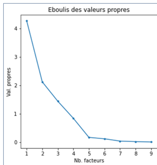
Figure 182 – Diagramme des valeurs propres – AFDM – Données "Autos 2005"
