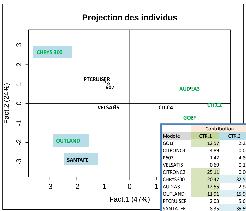
Figure 189 – Carte des individus illustrés selon leur contribution – AFDM – Données "Autos 2005"
