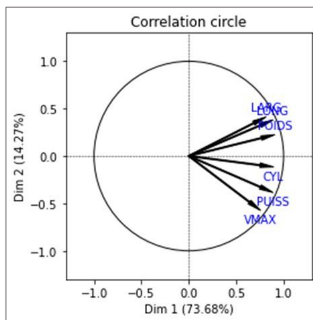
Figure 11 – Cercle des corrélations – Données "Autos"
