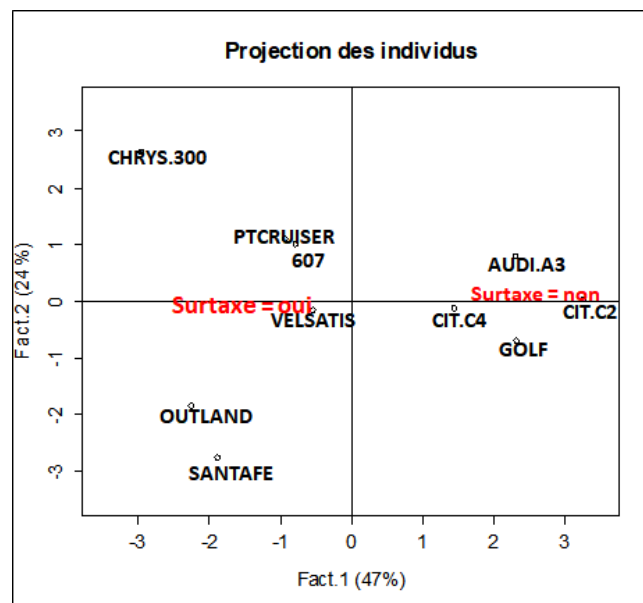
Figure 194 – Position des modalités supplémentaires – AFDM – Données "Autos 2005"
