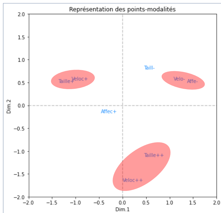
Figure 150 – Représentation des points modalités – ACM – Données "Canidés"
