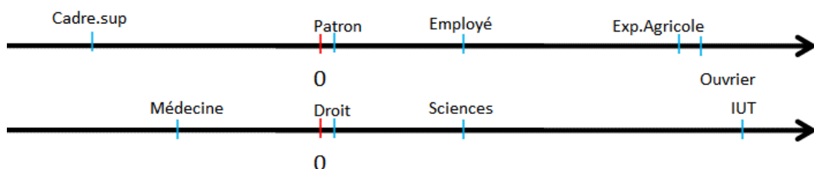
Figure 113 – Positions des modalités lignes et colonnes sur le 1 er facteur – Données "CSP Filières"
