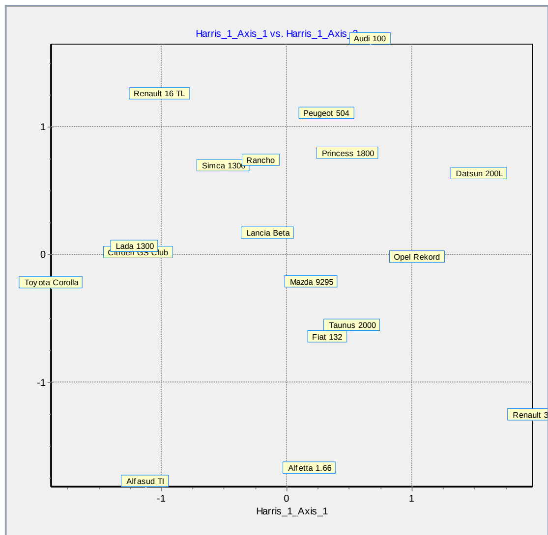
Figure 81 – Méthode de Harris – Carte des individus – Données "Autos bruitées"
