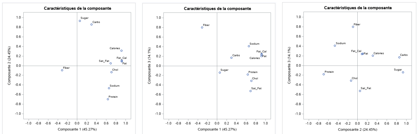
Figure 25 – Cercles des corrélations – SAS PRINCOMP – Données "Burger King"
