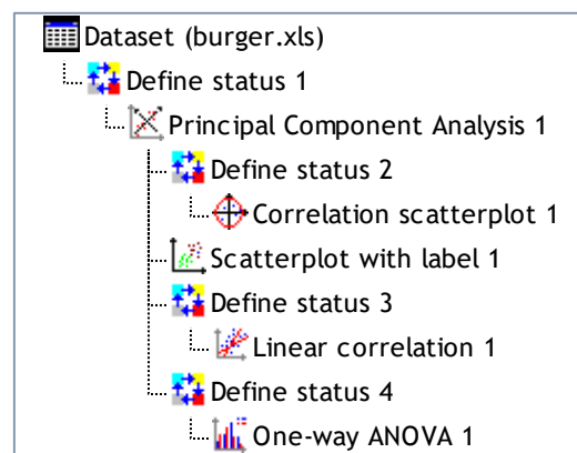
Figure 38 – Diagramme de traitements pour l'ACP – TANAGRA – Données "Burger King"
