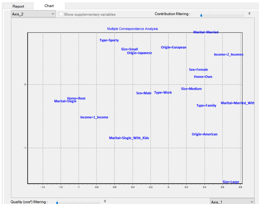
Figure 171 – Carte des modalités – ACM – TANAGRA – Données "Cars"
