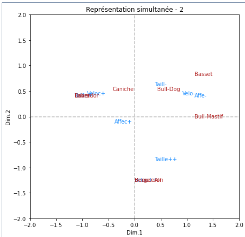
Figure 158 – Représentation simultanée 2 – ACM – Données "Canidés"
