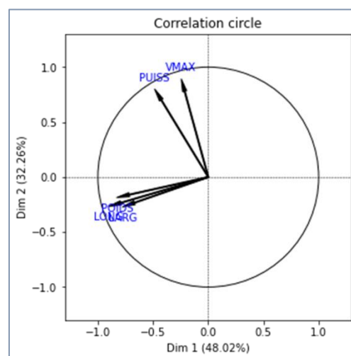
Figure 57 – Cercle des corrélations – ACP sur corrélations partielles
