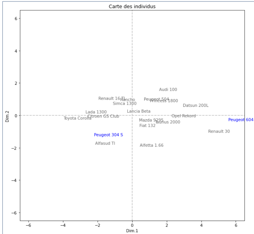
Figure 17 – Position des observations supplémentaires – Données "Autos"
