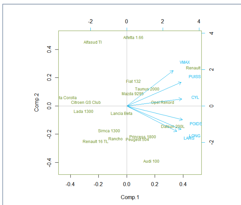
Figure 15 – Représentation "biplot" – Données "Autos"
