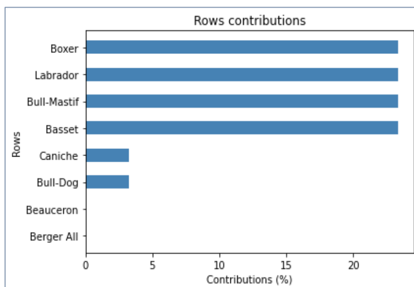
Figure 156 – Contributions des individus au 1er facteur – ACM – Données "Canidés"
