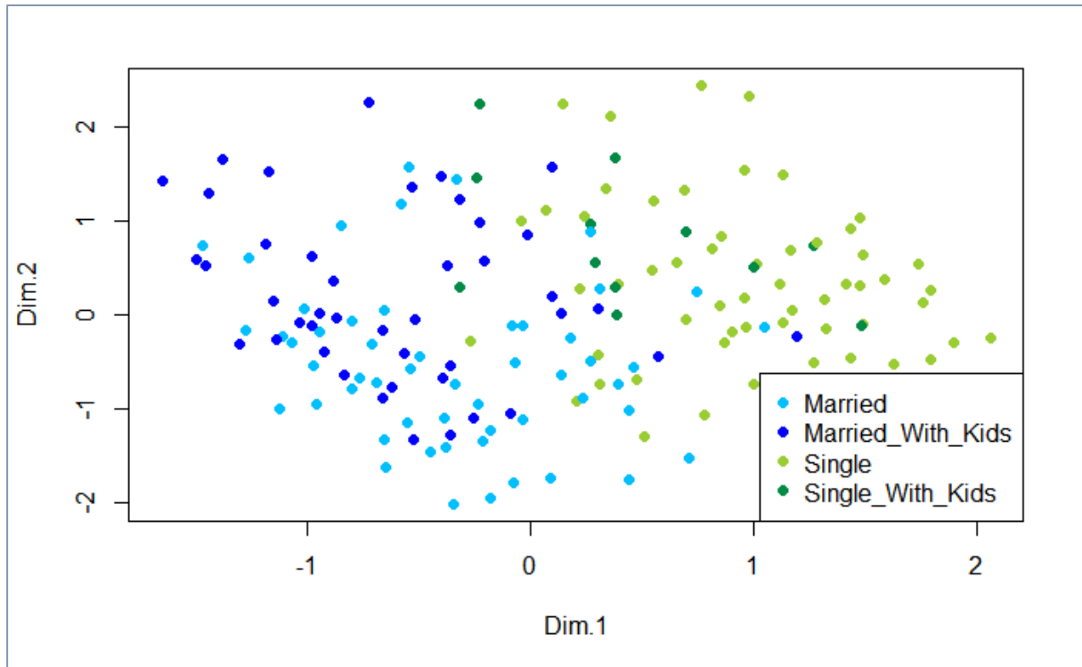
Figure 177 – Carte des individus – ACM – R, package "ca" – Données "Cars"
