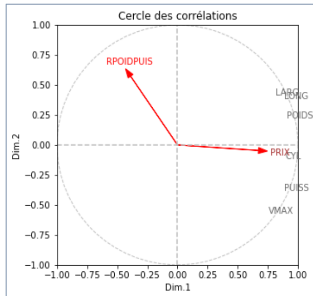
Figure 19 – Cercle des corrélations avec variables illustratives – ACP – Données "Autos"
