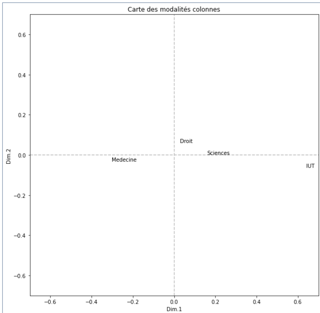
Figure 108 – Carte des modalités colonnes – 1er plan factoriel – Données "CSP Filières"
