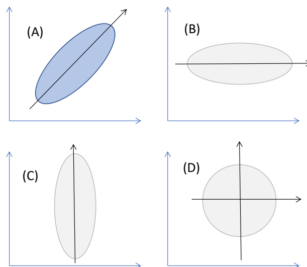
Figure 2 – Types de liens entre deux variables quantitatives
