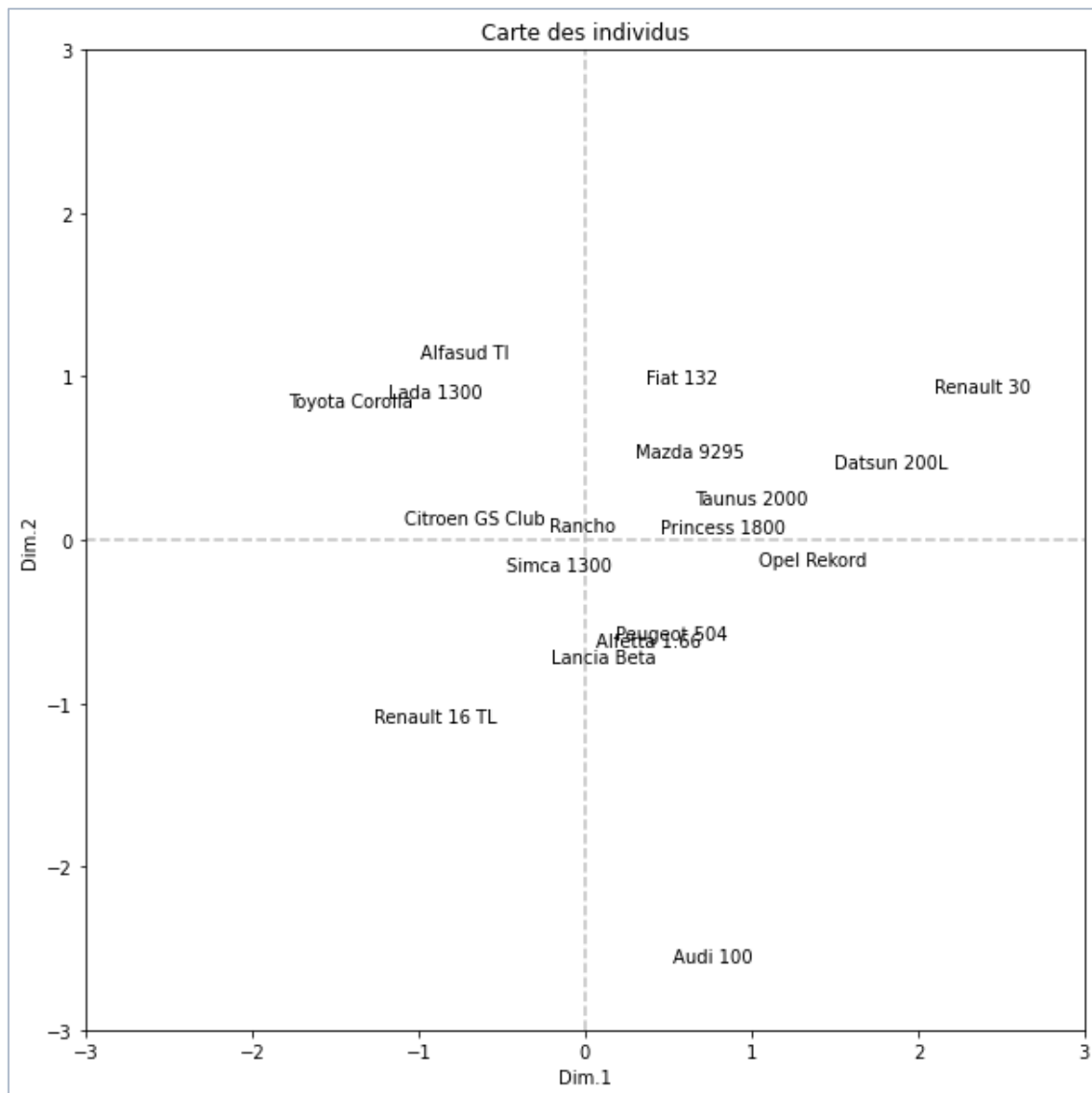
Figure 75 - Carte des individus - AFP - Données "Autos bruitées"
