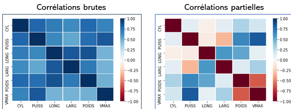
Figure 52 – Corrélations brutes et partielles – Données "Autos"
