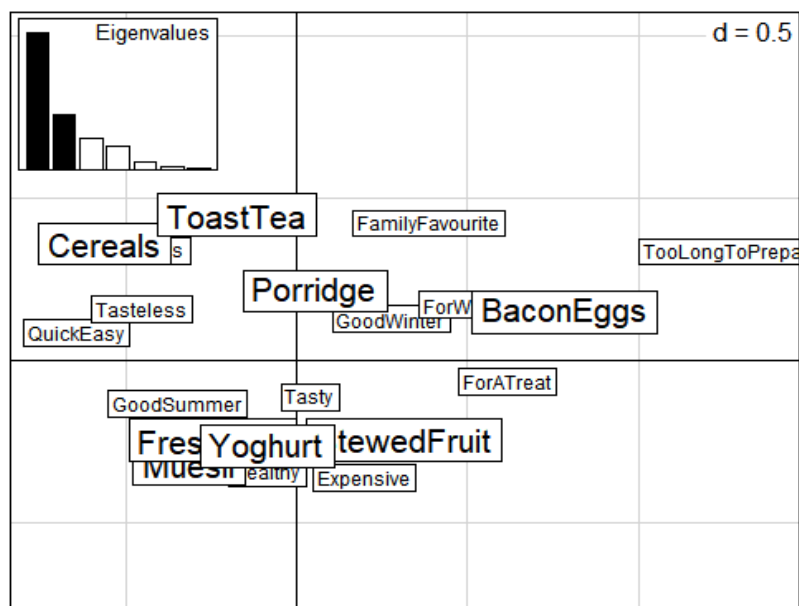
Figure 141 – Représentation simultanée – AFC – R, package "ade4"
