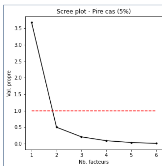
Figure 44 – Borne basse de l'intervalle de confiance bootstrap des v.p. – Données "Autos"
