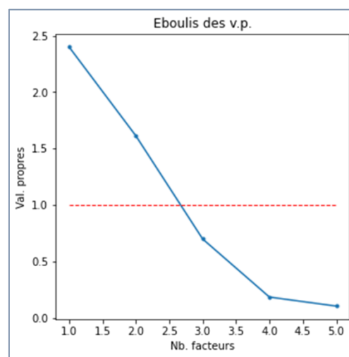
Figure 56 – Eboulis des v.p. – ACP sur corrélations partielles
