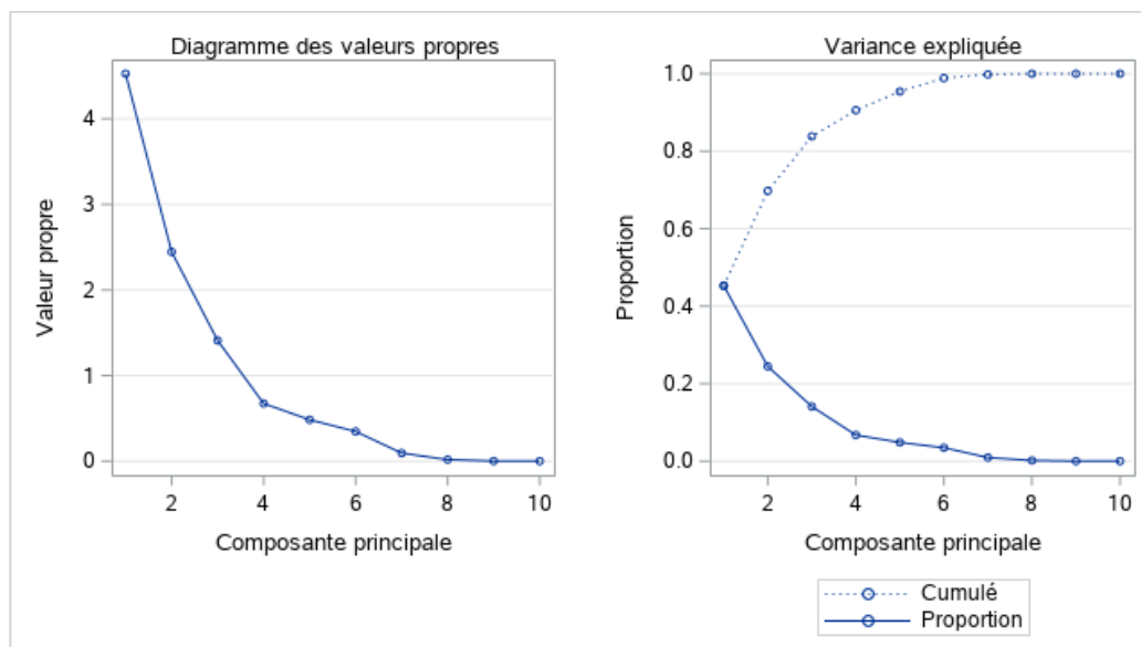
Figure 23 – Eboulis des valeurs propres et évolution de la variance expliquée – SAS PRINCOMP – Données "Burger King"
