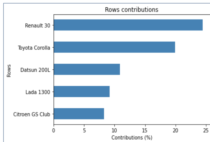
Figure 14 – 5 plus fortes contributions au premier facteur de l'ACP – Données "Autos"
