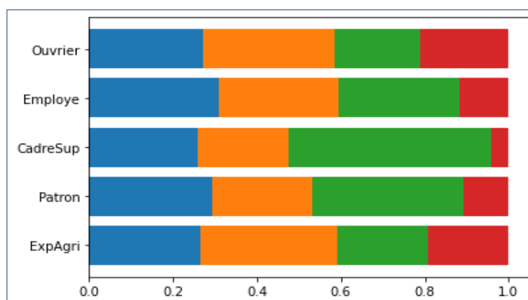
Figure 101 – Structure des choix de filières selon les CSP – Données "CSP – Filières"
