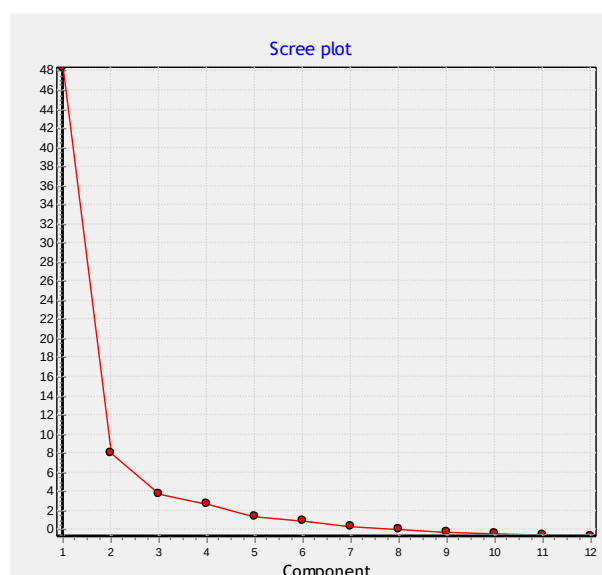
Figure 77 – Méthode de Harris – Eboulis des valeurs propres – Données "Autos bruitées"
