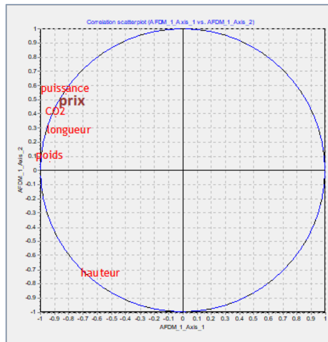
Figure 193 – Variable supplémentaire "Prix" dans le cercle des corrélations – AFDM – Données "Autos 2005"
