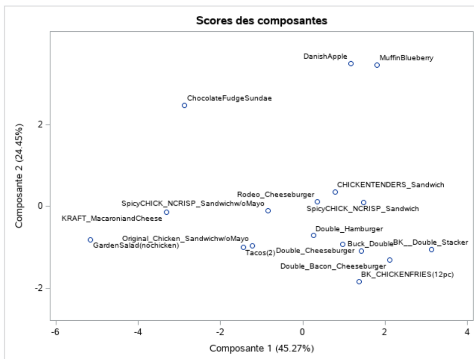
Figure 26 – Carte des individus premier plan factoriel – SAS PRINCOMP – Données "Burger King"
