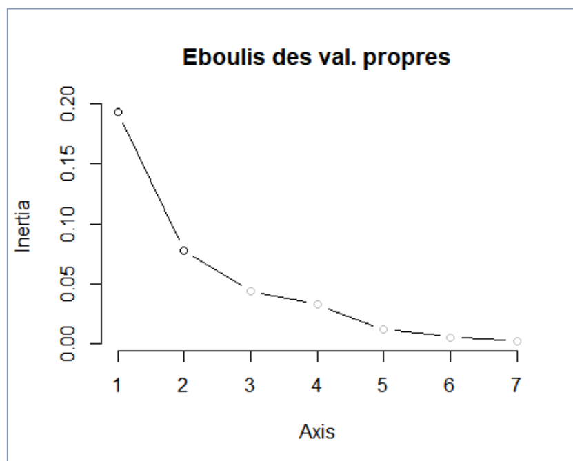
Figure 139 – Eboulis des valeurs propres – AFC – R, package "ade4"
