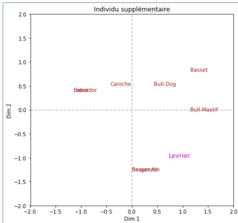
Figure 159 – Individu supplémentaire – ACM – Données "Canidés"
