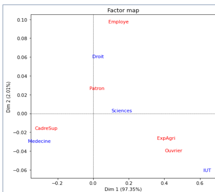
Figure 116 – Représentation simultanée "fanalysis" – AFC – Données "CSP Filières"
