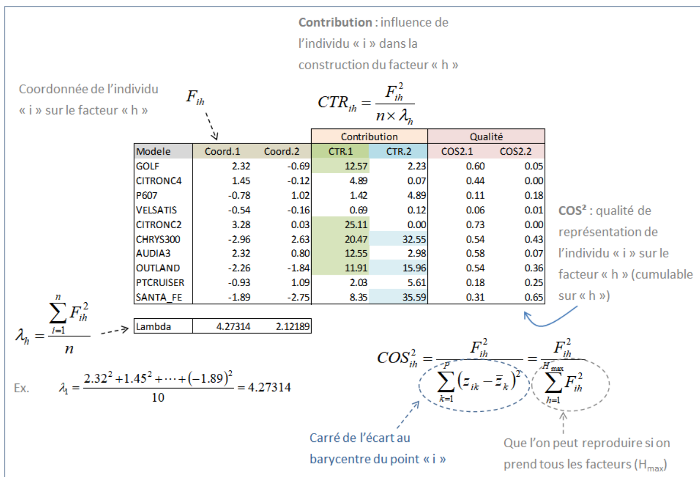
Figure 188 – Coordonnées des individus et aides à l'interprétation – AFDM – Données "Autos 2005"
