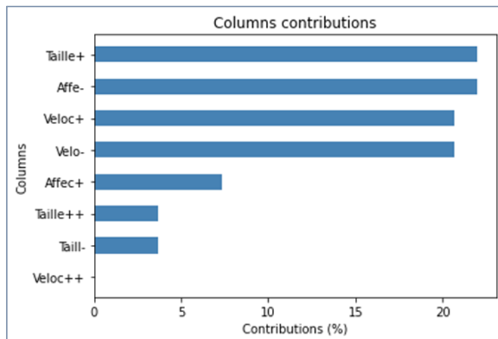
Figure 153 – Contributions des points-modalités sur le 1 er facteur – ACM – Données "Canidés"
