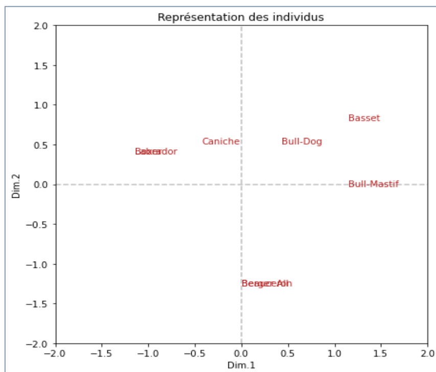
Figure 155 - Représentation des individus - ACM - Données "Canidés"
