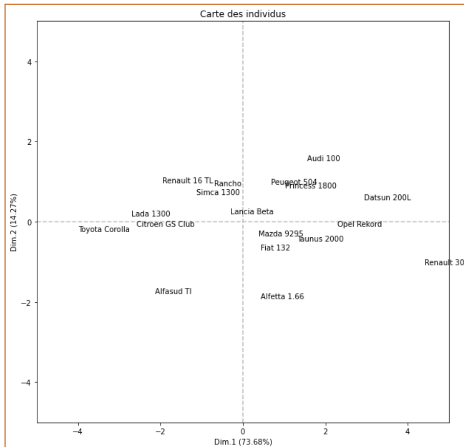
Figure 13 – Carte des individus – Version 2 – Données "Autos"
