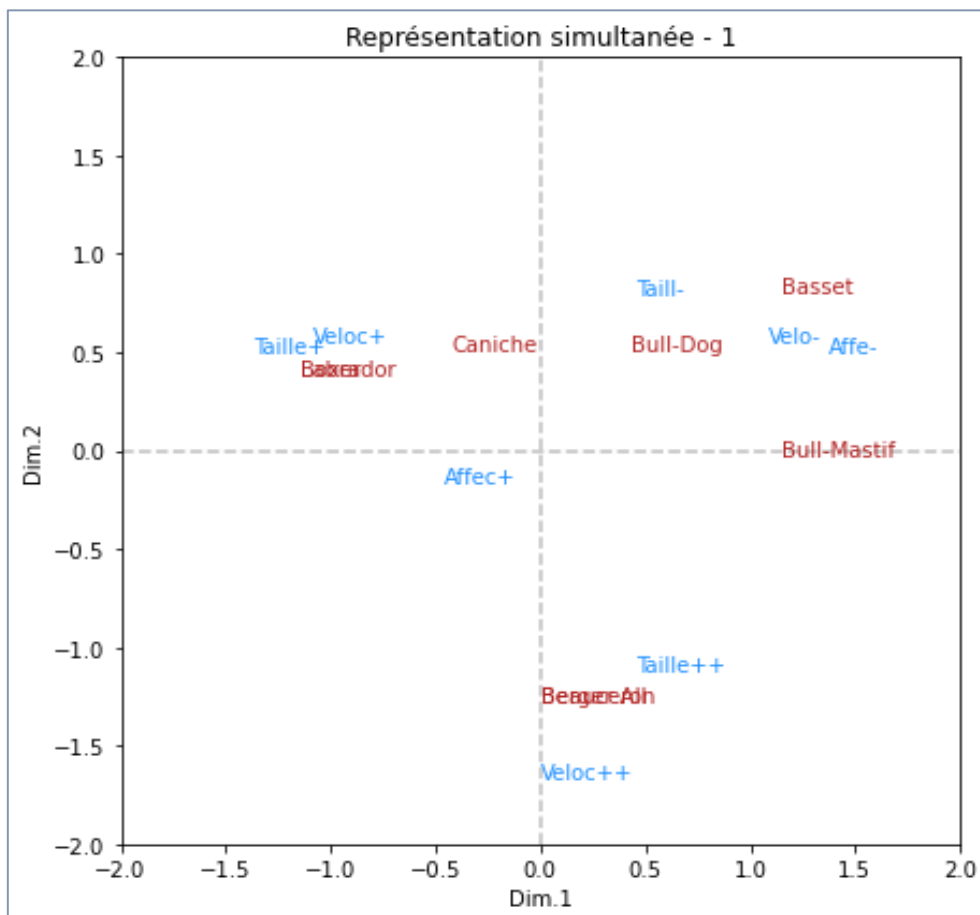
Figure 157 – Représentation simultanée 1 – ACM – Données "Canidés"
