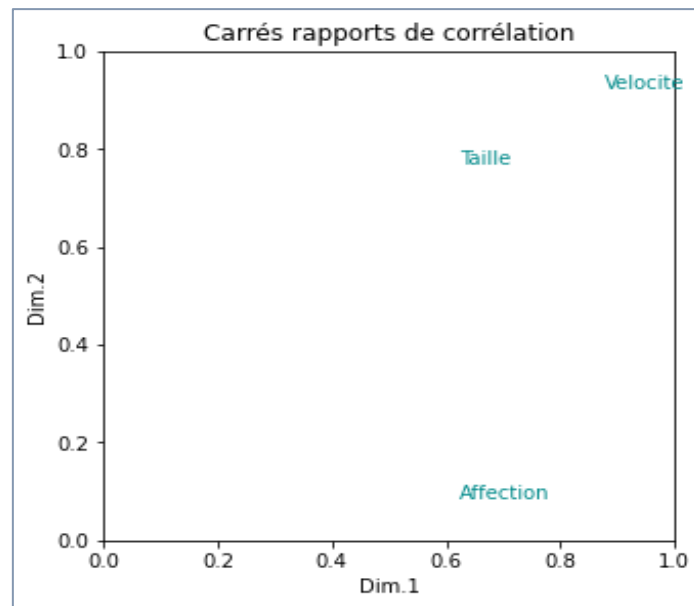
Figure 154 – Représentation des carrés des rapports de corrélation des variables – ACM – Données "Canidés"
