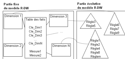
FIG. 1 – Modèle R-DW .
