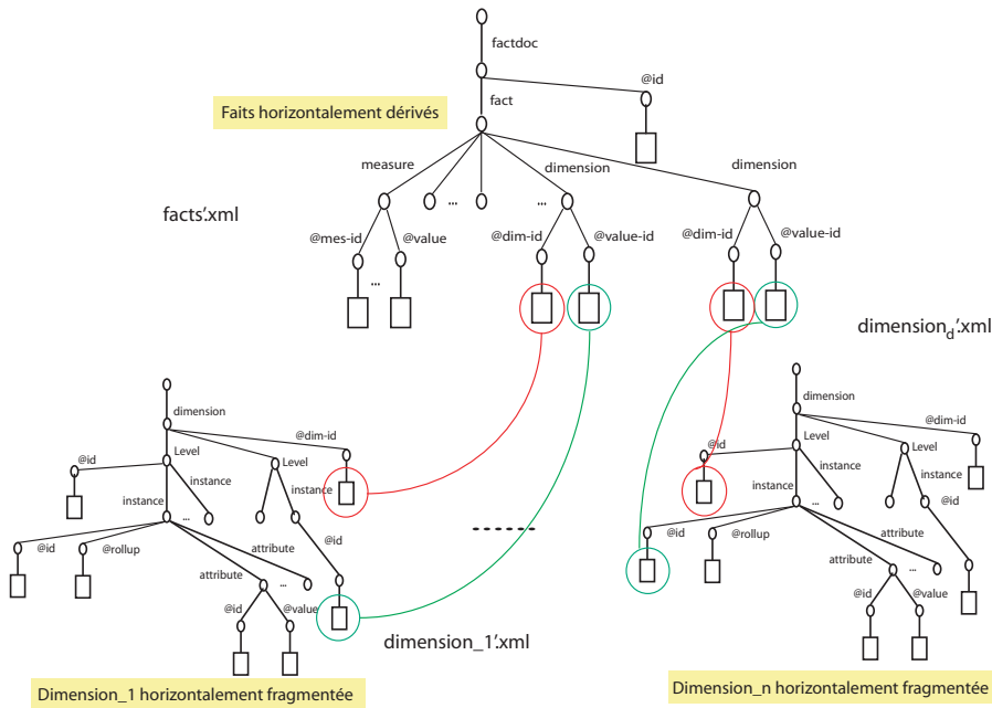
FIG. 5 – Exemple de fragment d'entrepôt de données XML
